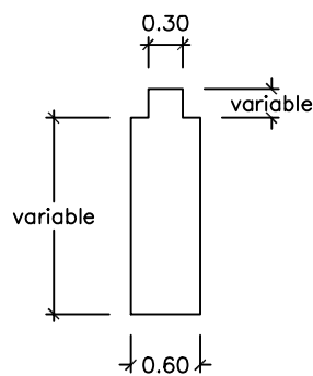
SECCIÓN
