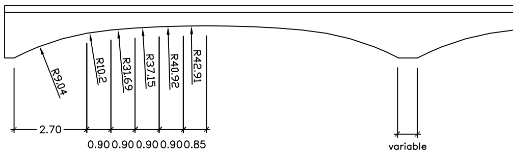
ALZADOS
