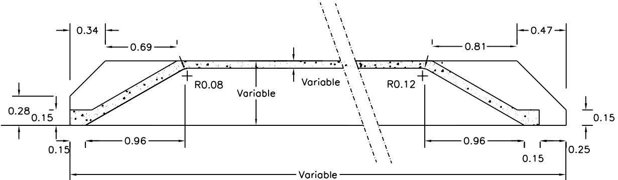
SECCION TRANSVERSAL
