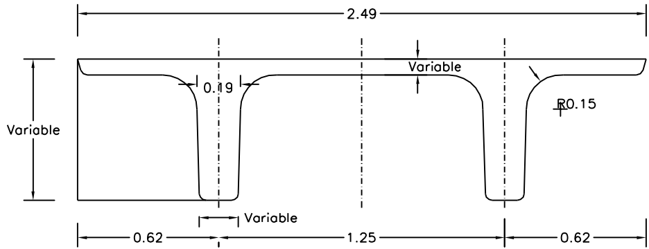
SECCION TRANSVERSAL
